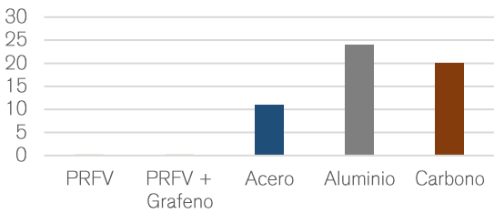
Conductividad termica
